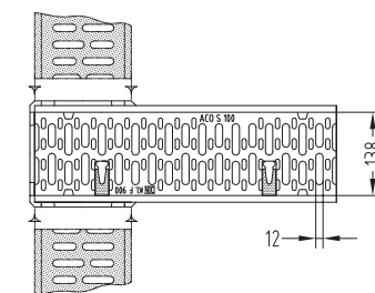
Parte superior sumidero - Parte superior do sumidouro
