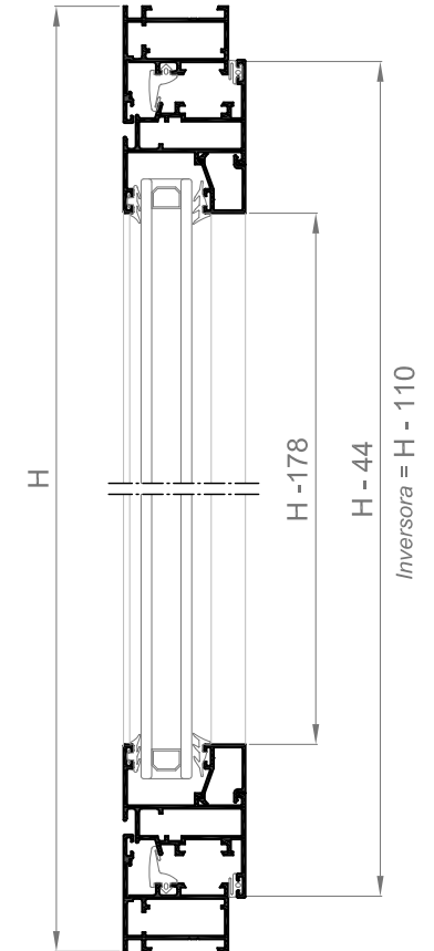
Sección B-B'
