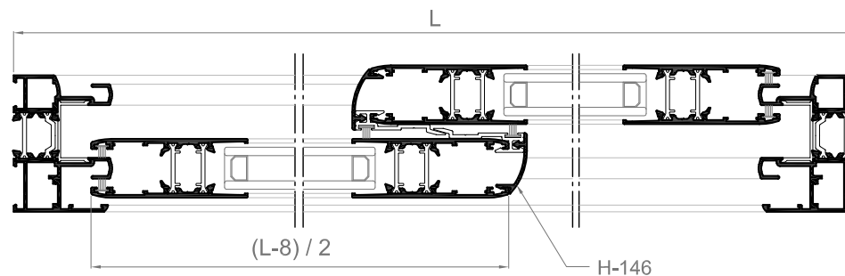
Sección A-A'
