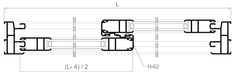
Sección A-A'
