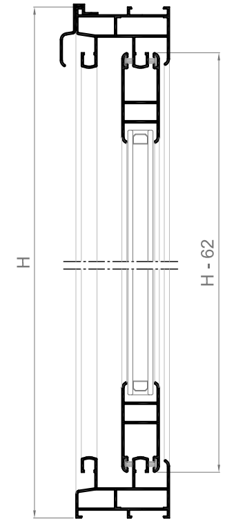
Sección B-B'
