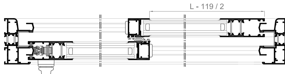
Sección A-A' / Hoja Minimalista
