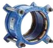
Serie 621/10 Unión Supa Plus™ Anti-tracción para tuberías de PE y PVC Fundición dúctil DN 32-300 PN 16
