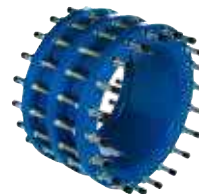
Serie 265/50 Carrete de desmontaje Con brida central Acero DN 50-2000 PN 10/16/25
