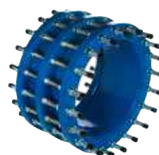
Serie 265/50 Carrete de desmontaje fabricado para todos los materiales de tubería con brida central Acero DN 50-2200 PN 10/16/25
