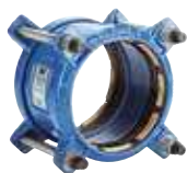
Serie 621/10 Supa Plus™ Unión recta antitracción para las tuberías de PE y uPVC Fundición dúctil DN 32-300 PN 16
