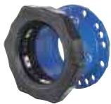
Serie 633 Supa Maxi™ Brida enchufe universal y antitracción para todas las tuberías. Taladro de brida universal Fundición dúctil DN 40-400 PN 10/16
