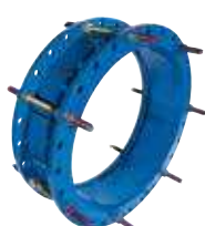
Serie 265/30 Carrete de desmontaje fabricado para todos los materiales de tubería Acero DN 300-1200 PN 10/16/25
