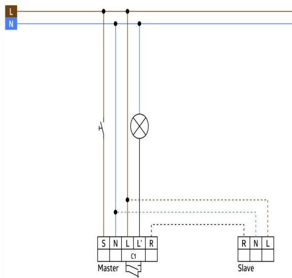
Esquemas de conexión
