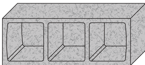
CASETÓN HORMIGÓN MODELO R.H.
