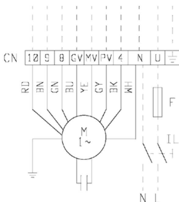
» Esquema eléctrico FWB-C 05-06-08-10-11 7 velocidad
