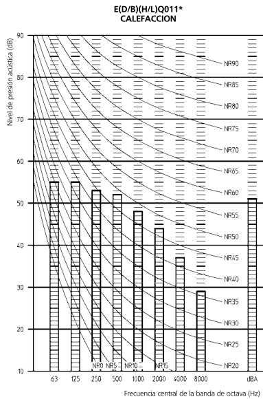
EBHQ011-016BB6V3
