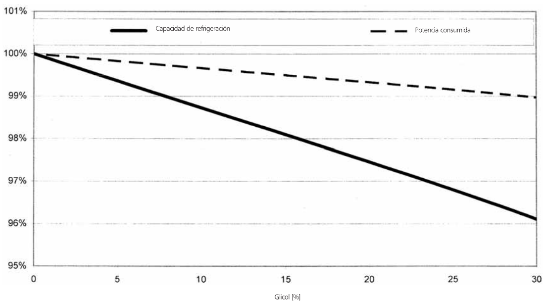
EBHQ011-016BB6V3
