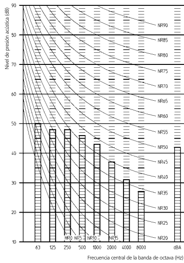
E(D/B)(H/L)Q014* CALEFACCION
