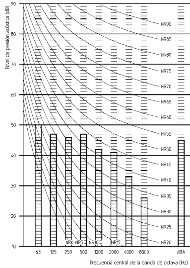
E(D/B)(H/L)Q014* REFRIGERACIÓN
