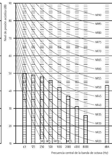
E(D/B)(H/L)Q016* CALEFACCION
