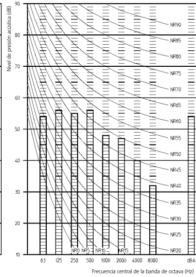
E(D/B)(H/L)Q016* REFRIGERACIÓN
