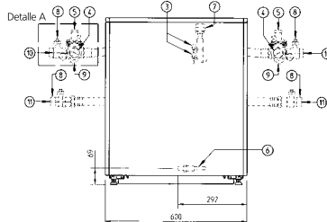
Detalle A
