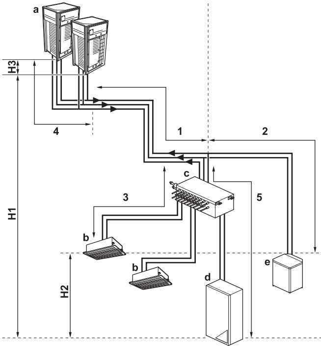
Conexión con unidades VRV DX y cajas hidráulicas
