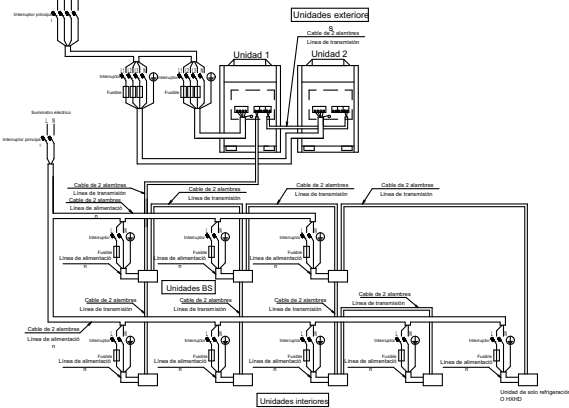
La fuente de alimentación se suministra a cada unidad exterior individualmente.
