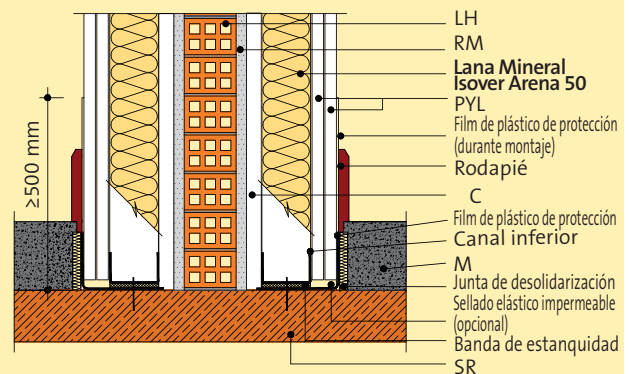
Solución sobre suelos flotantes - solución con una hoja de fábrica, mixta:
