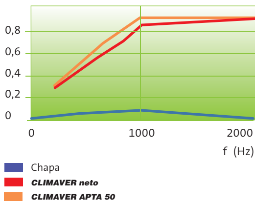
Coeficiente de absorción, \alpha_s
