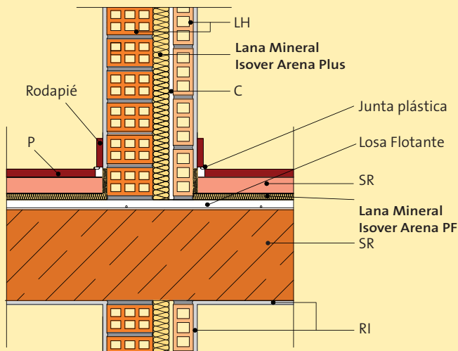
Solución sobre suelos flotantes - solución con hojas de fábrica, mixta:
