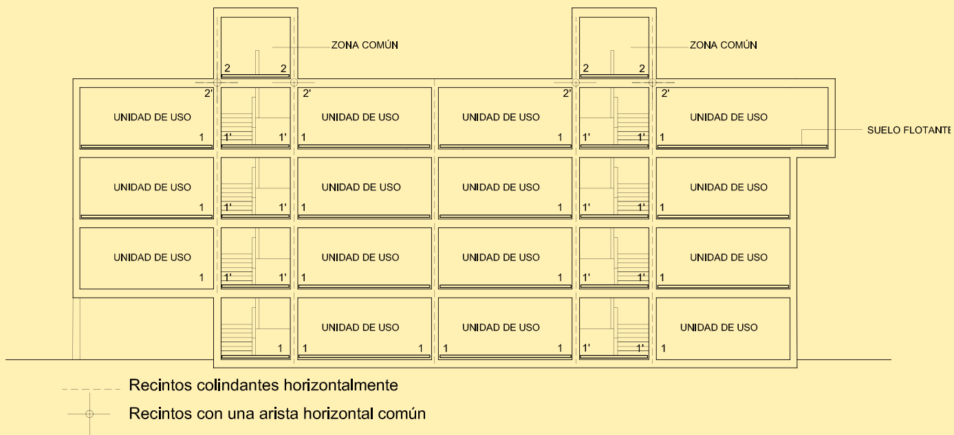
Figura de disposición de suelos flotantes para limitar la transmisión de ruido de impactos entre recintos colindantes horizontalmente (1-1') y entre recintos con una arista horizontal común (2-2').
