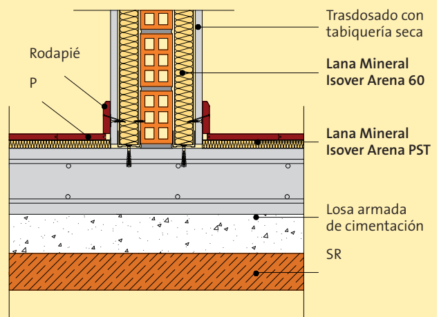
Solución sobre suelos flotantes - solución con una hoja de fábrica, mixta:
