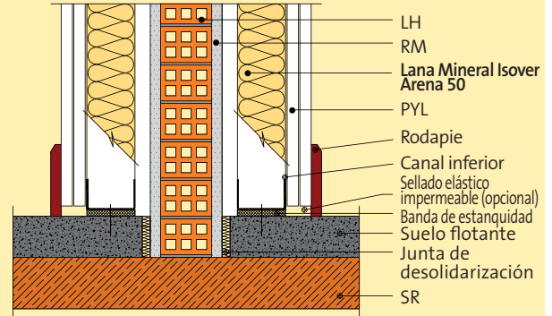
Solución sobre capa de compresión - solución mixta:
