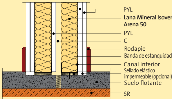
Solución sobre capa de compresión - solución PYL:
