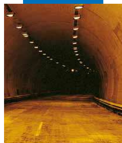
Aplicación por proyección de Planiseal 88 blanco en un túnel
