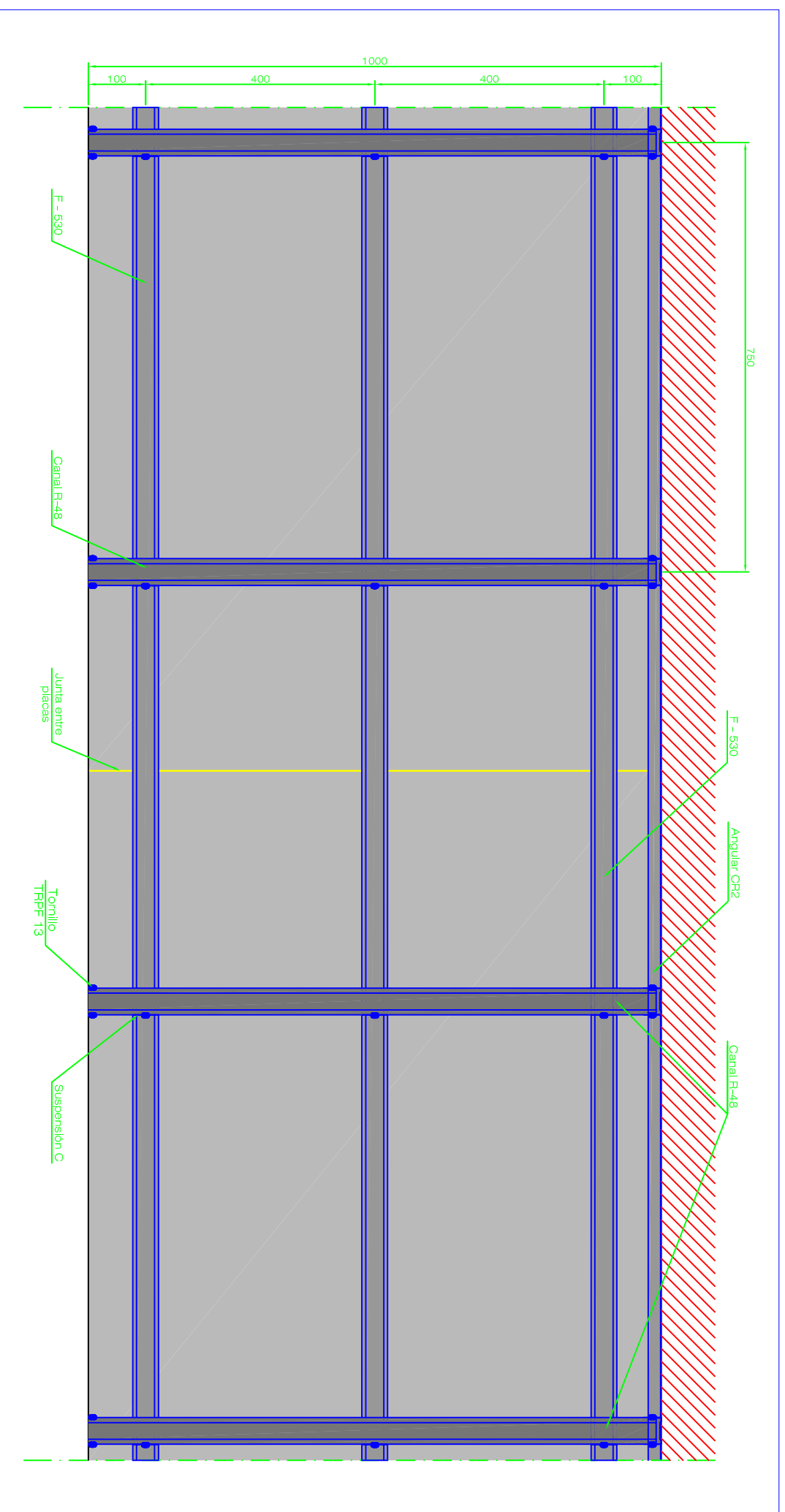
Planta E 1-100
