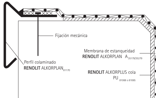
Fig. 3: Encolado en la totalidad de la membrana RENOLIT ALKORPLAN A
