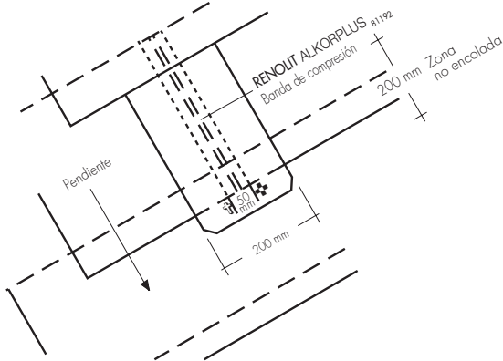
Fig. 2: Junta entre final de rollos
