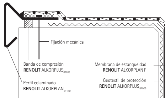
Fig. 4: Estanqueidad contra el viento, por puesta en obra en independencia de otras membranas RENOLIT ALKORPLAN
