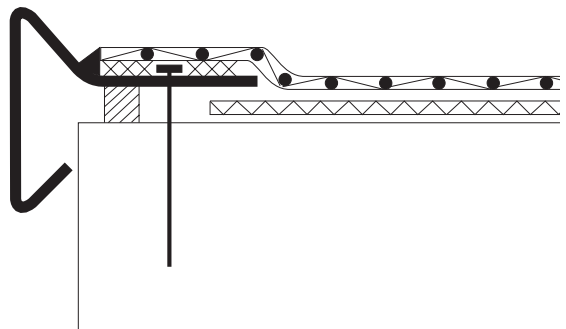
Fig. 2 Utilización de junta de compresión RENOLIT ALKORPLUS 81058
