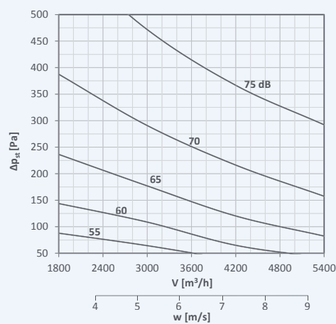
400x400
