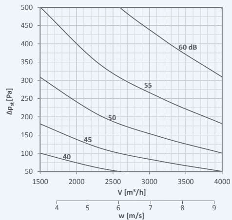
600x200
