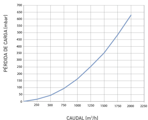
PERDITE DI CARICO MODULO SimeConn Multi \varnothing 3/4" - DN 18 SOLO NUCLEO IDRAULICO
