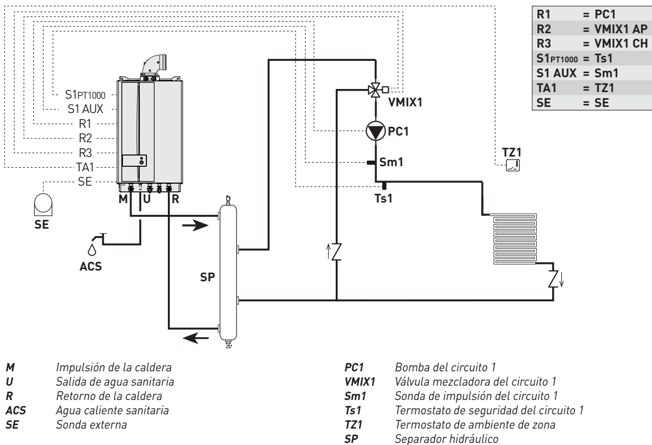
Tipo 2: Instalación con un circuito mezclado multizona
