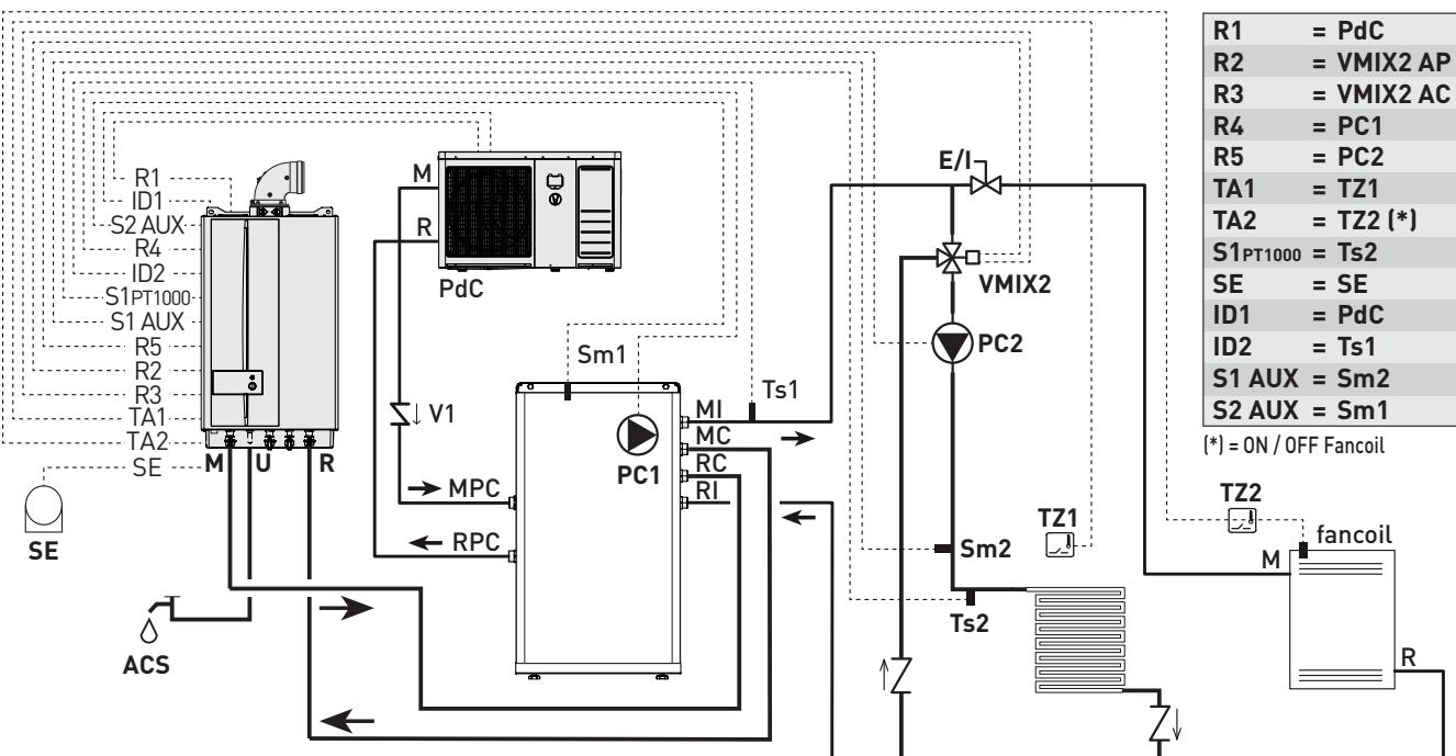
Tipo 14: Instalación con un circuito mezclado multizona y una instalación de gestión de calor/frío
