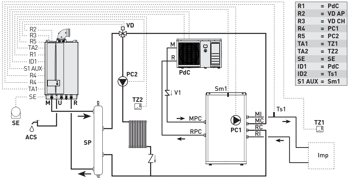
Tipo 12: Instalación con un circuito directo multizona y una instalación de gestión de calor/frío
