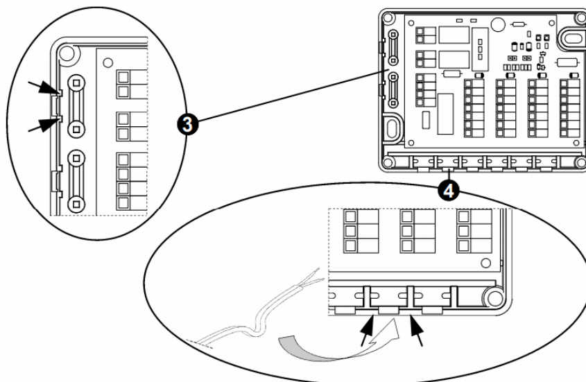
Fig. 3: Istruzioni passaggio cavi / Cable entry instructions / Instructions pour le passage des câbles / Instrucciones paso de cables. Abb. 3: Einführung der Kabel.
