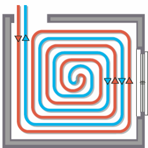
Sistema espiral
