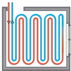
Sistema doble serpentin
