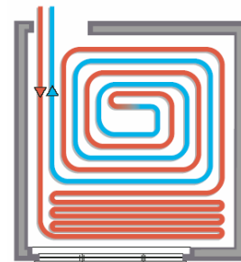
Circuito con zonas frías
