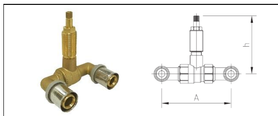
Válvula MultiStandard Plus en "U"
