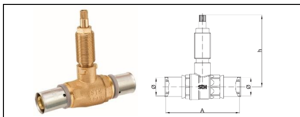
Válvula MultiStandard Plus
