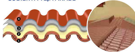
CUBIERTA TEJA ÁRABE
