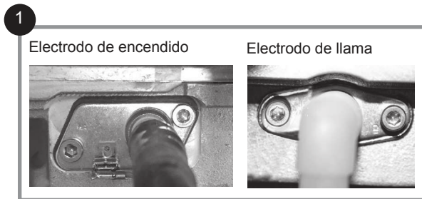
figura 45 - Electrodo de detección de llama
