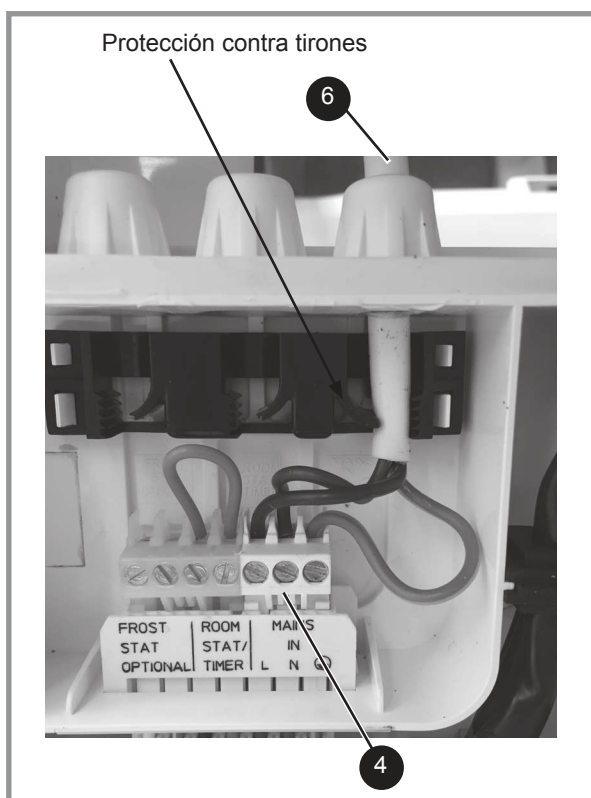
figura 33 - Cable de red preinstalado
