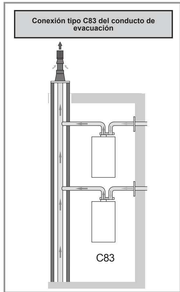
figura 25 - Posibilidades de conexión (instalación tipo C83)
