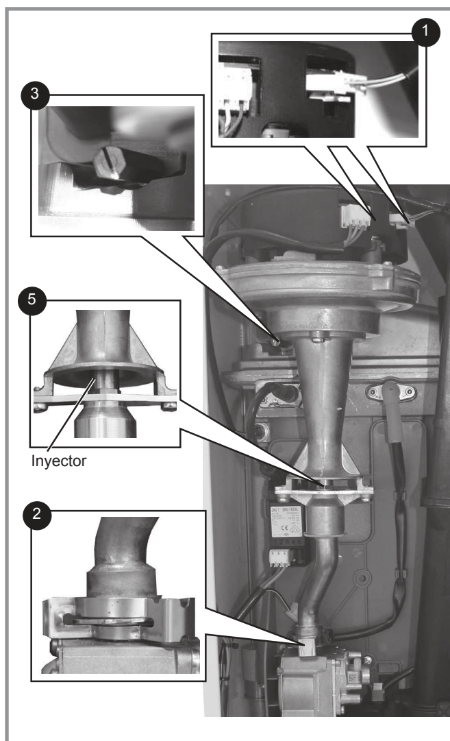
figura 40 - Retirada del ventilador y del tubo Venturi
