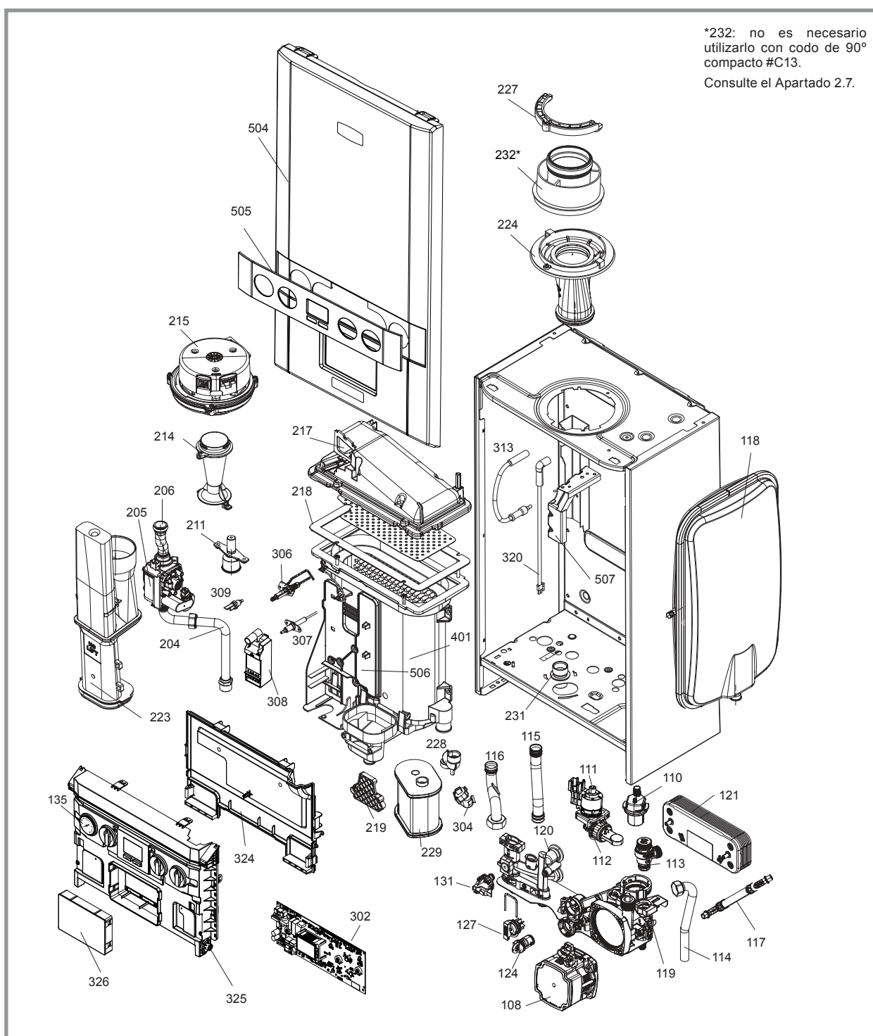
figura 4 - Ensamblaje de la caldera
