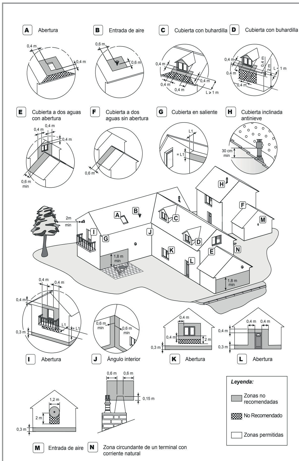
figura 27 - Normas para instalar los terminales sellados de una caldera de gas (tipos C13, C33, C43)
