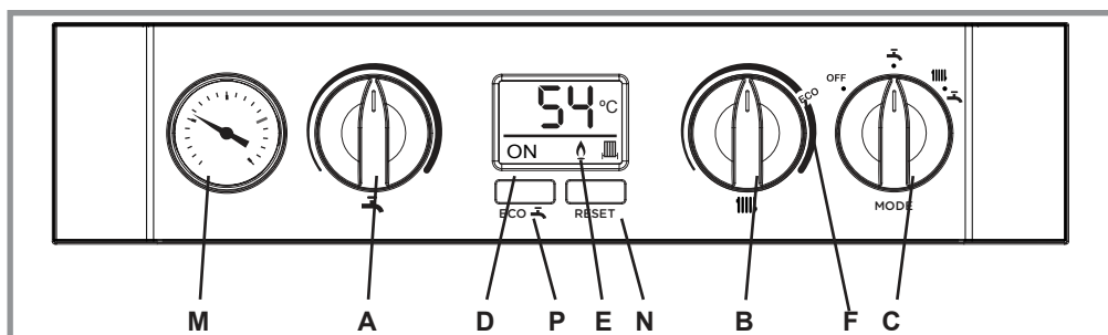
figura 35 - Controles de funcionamiento
