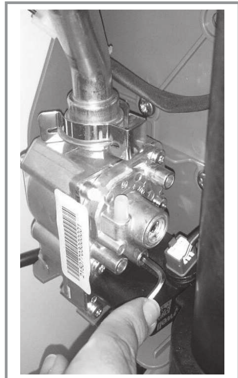
figura 34 - Entrada de presión del gas
