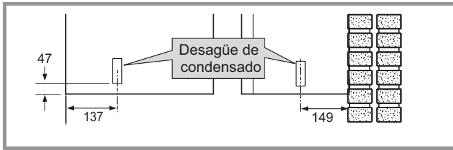
figura 28 - Ubicación del tubo de desagüe del agua de condensación
