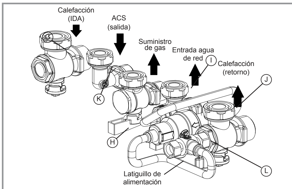
figura 36 - Conexiones de tubería
