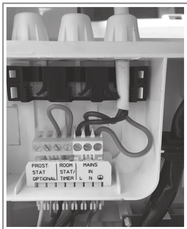
figura 31 - Conexiones preinstaladas (lado izquierdo)
