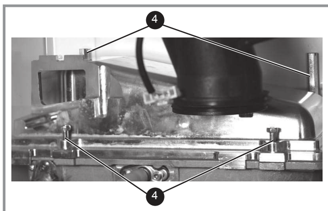
figura 42 - Retirada del quemador
