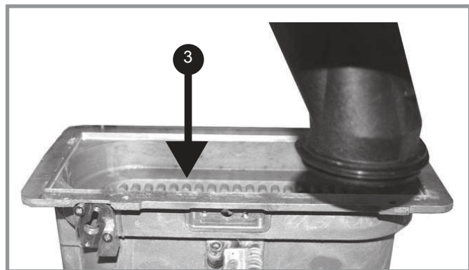
figura 46 - Intercambiador de calor
