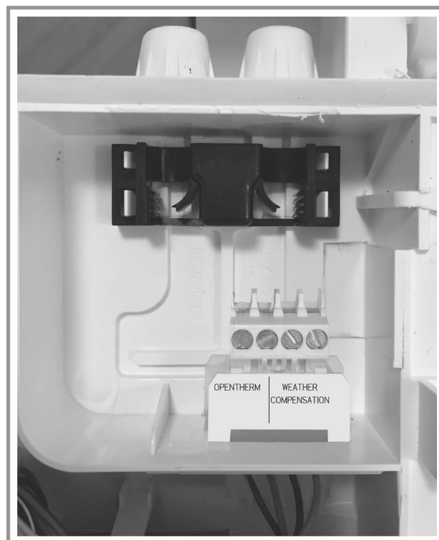
figura 32 - Conexiones preinstaladas (lado derecho)
