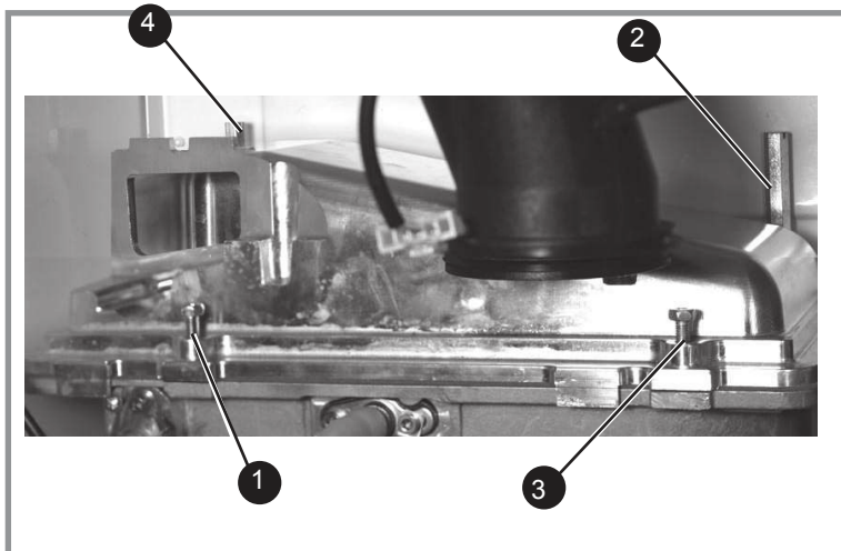
figura 47 - Reensamblaje del colector del conducto de evacuación
