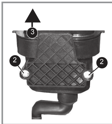
figura 41 - Retirada del colector
