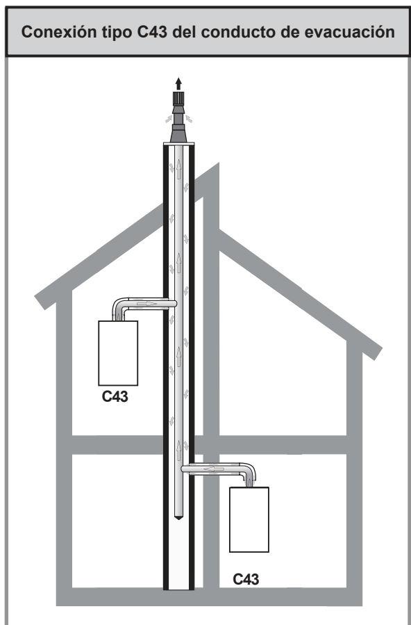
figura 21 - Posibilidades de conexión (tipo C43)
