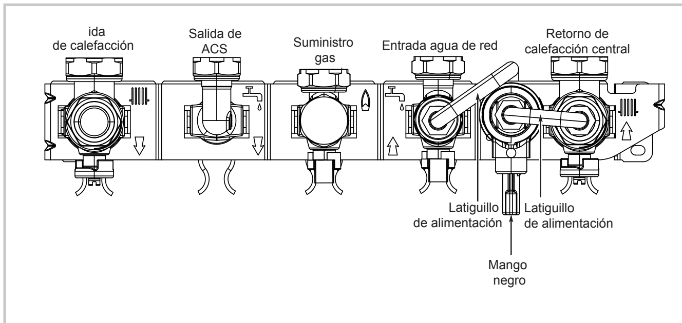
figura 30 - Conexiones del latiguillo de alimentación
