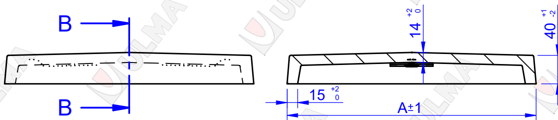
CORTE B-B
