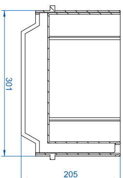
DETALLE A
