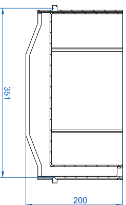
DETALLE A
