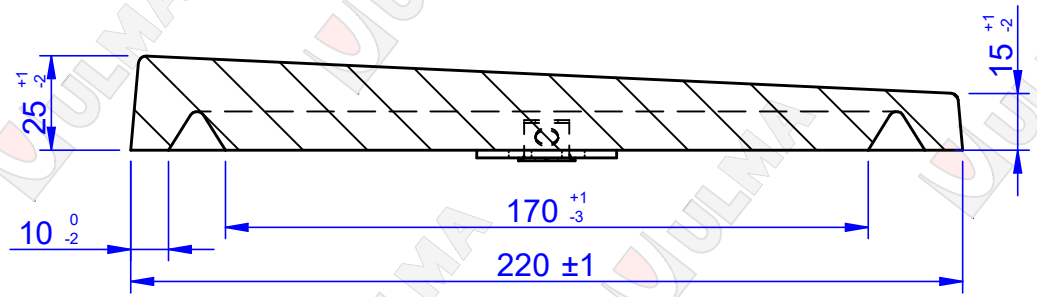
CORTE A-A 1:2
