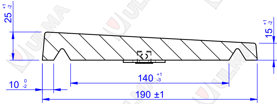
CORTE A-A 1:2
