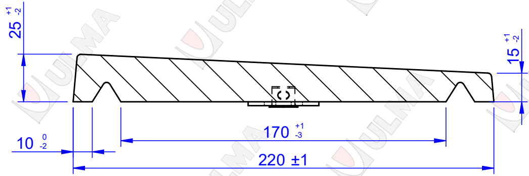
CORTE A-A 1:2
