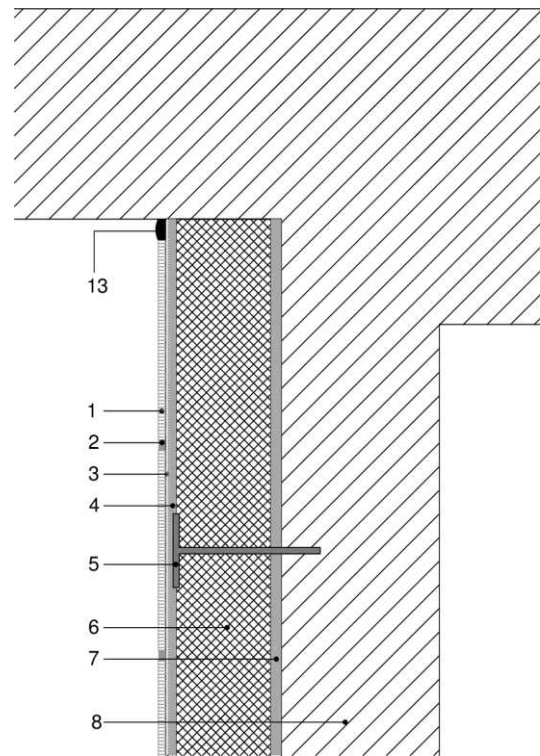
Figura 5.3d: Coronación. Encuentro con cubierta plana.
