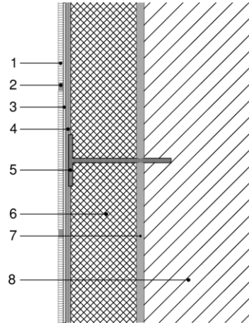
Figura 5.1: Sección vertical / horizontal.
