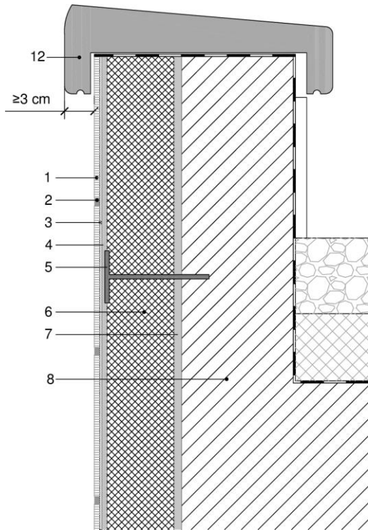
Figura 5.3a: Coronación con pieza pétreo.
