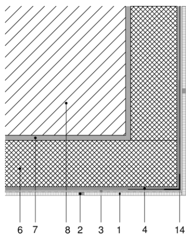
Figura 5.8a: Esquina saliente.
