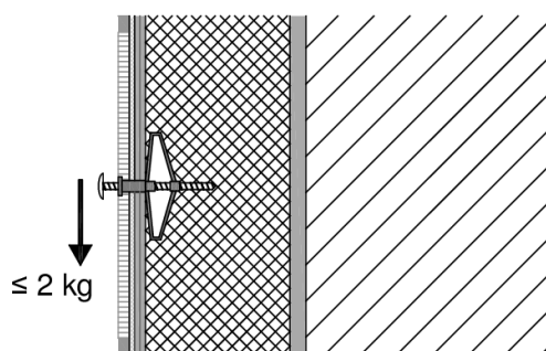
Figura 5.9: Anclaje para cargas ligeras con tacos para pared hueca.
