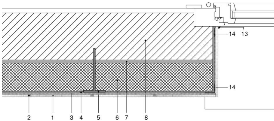
Figura 5.6b: Jamba sin aislamiento.
