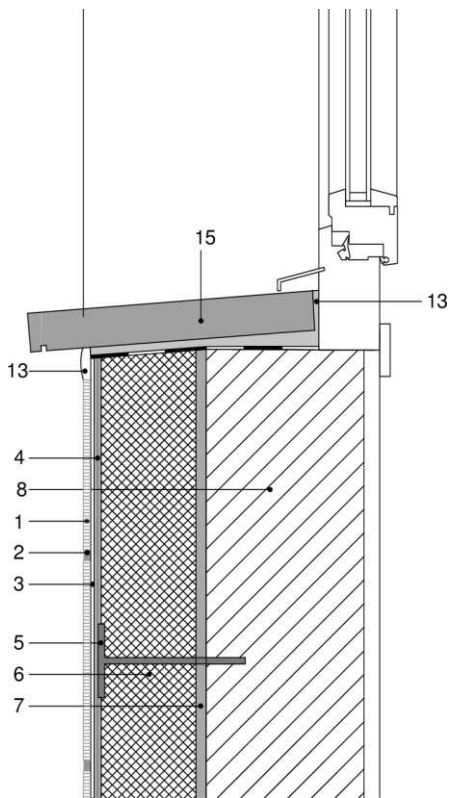
Figura 5.5a: Antepecho con vierteaguas pétreo.
