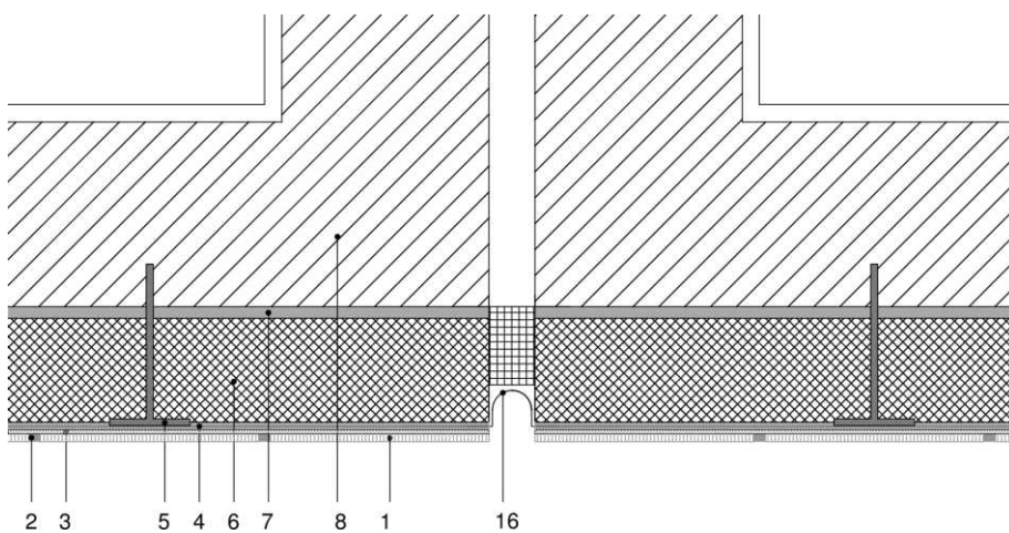
Figura 5.7: Junta de dilatación.
