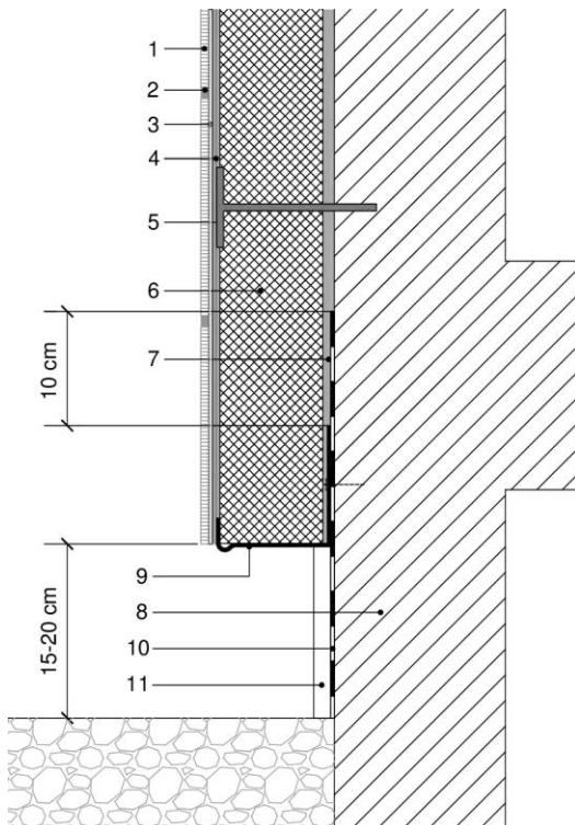
Figura 5.2a: Arranque desde suelo.
