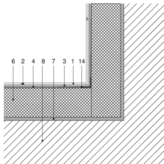
Figura 5.8b: Esquina entrante.
