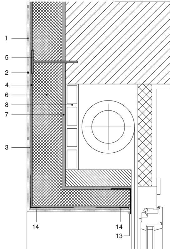
Figura 5.4b: Dintel con caja de persiana.
