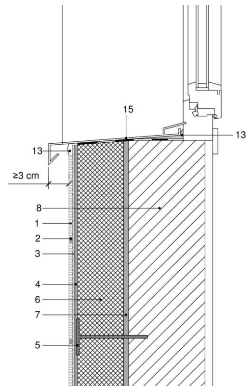
Figura 5.5b: Antepecho con vierteaguas metálico.
