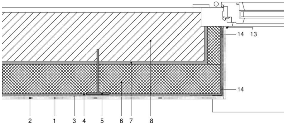
Figura 5.6a: Jamba con aislamiento.
