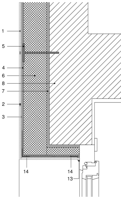
Figura 5.4a: Dintel.
