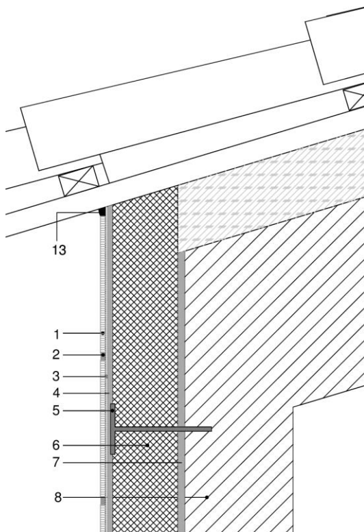
Figura 5.3c: Coronación. Encuentro con cubierta inclinada.
