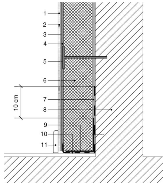
Figura 5.2b: Arranque en balcones.
