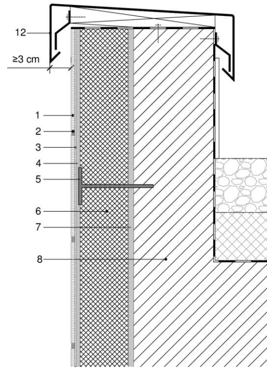
Figura 5.3b: Coronación con pieza metálica.
